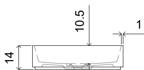
versione marmo CUBA02 Marble Product CUBA02
