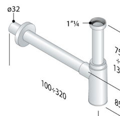
Sifone per scarico a muro in ottone Siphon for wall drain in brass
