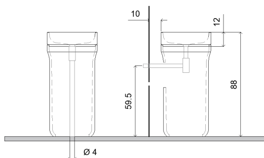
Versione scarico a terra Floor drain version
