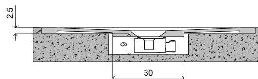
Versione incasso Recessed version
