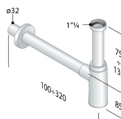
Sifone per scarico a muro in ottone Siphon for wall drain in brass
